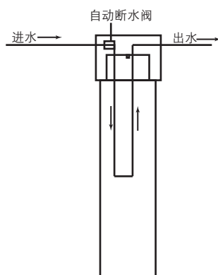
沸石活性炭折叠膜复合滤芯
