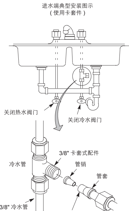
(图 1) 管路装置图
